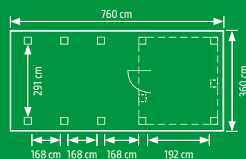
„Nürnberg Modern 2“ mit Geräteraum
